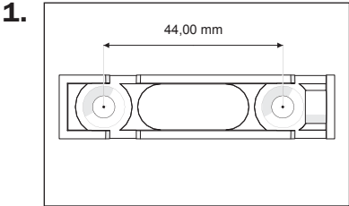
Bohrschablone für MMD.
