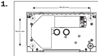
Bohrschablone für MMW.
