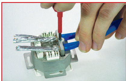
Mittels Schraubendreher den Bügel festschrauben. / Fix cable clip by use of a screwdriver.
