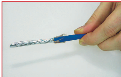
Das Schirmgeflecht auf ca. 2cm kürzen und über den Mantel zurückschieben. / Cut back Braid to 2cm and fold back over cable sheet.
