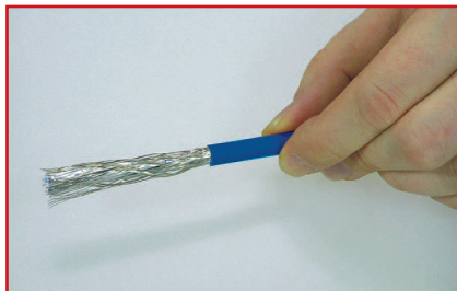
Kabel ca. 6cm absetzen. / Strip of jacket 6 cm.
