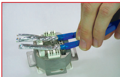
Die Kabel an der Dose ansetzen. / Put cables to the outlet.
