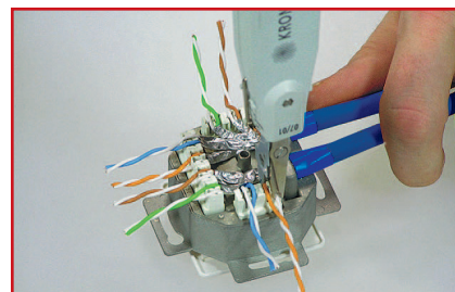
Die einzelnen Adern mit LSA Werkzeug (Art. Nr.: HKRONELSA) aufschalten. / Apply wires by use of LSA-Tool (Order Code: HKRONELSA). Cut off excess length.
