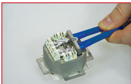
Dose fertig beschaltet. / Outlet with applied wires.
