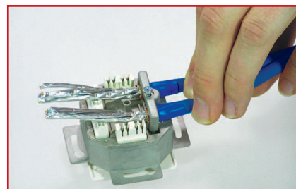
Den Bügel zur Befestigung der Kabel aufsetzen. / Put cable clip ready for fixing of cables.
