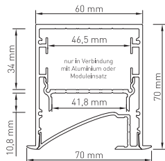
Aluminium Profil SLW glatt im SLT Profil mit Einsatz Aluminium profile SLW smooth in SLT profile with inset
