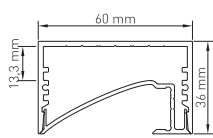
Aluminium Profil SLW glatt im SLA Profil Aluminium profile SLW smooth in SLA profile
