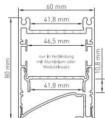
Aluminium Profil SLW glatt im SLH Profil mit Einsatz Aluminium profile SLW smooth in SLH profile with inset
