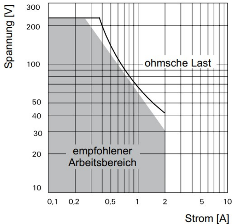
Lastkurve der Signalrelais (AC/DC)
