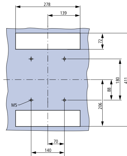
Aufbau der Montageplatte
